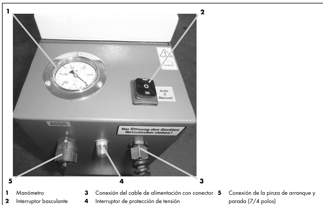
Fig. 6 Elementos de mando
