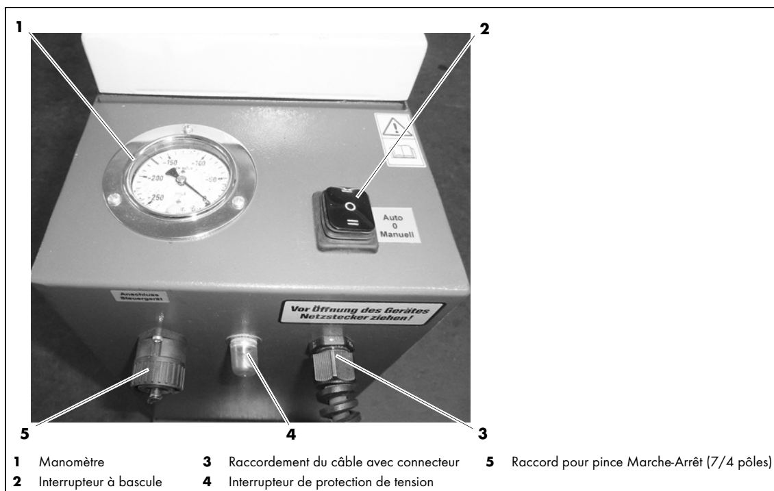
Fig. 6 Eléments de commande
