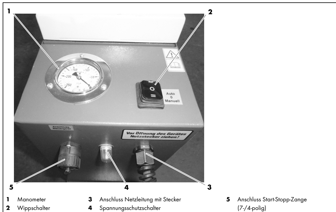
Abb. 6 Bedienelemente
