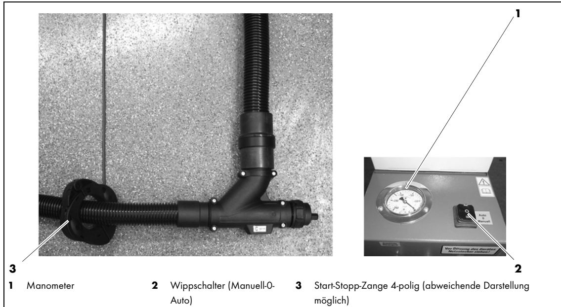
Abb. 5 Start-Stopp-Zange
