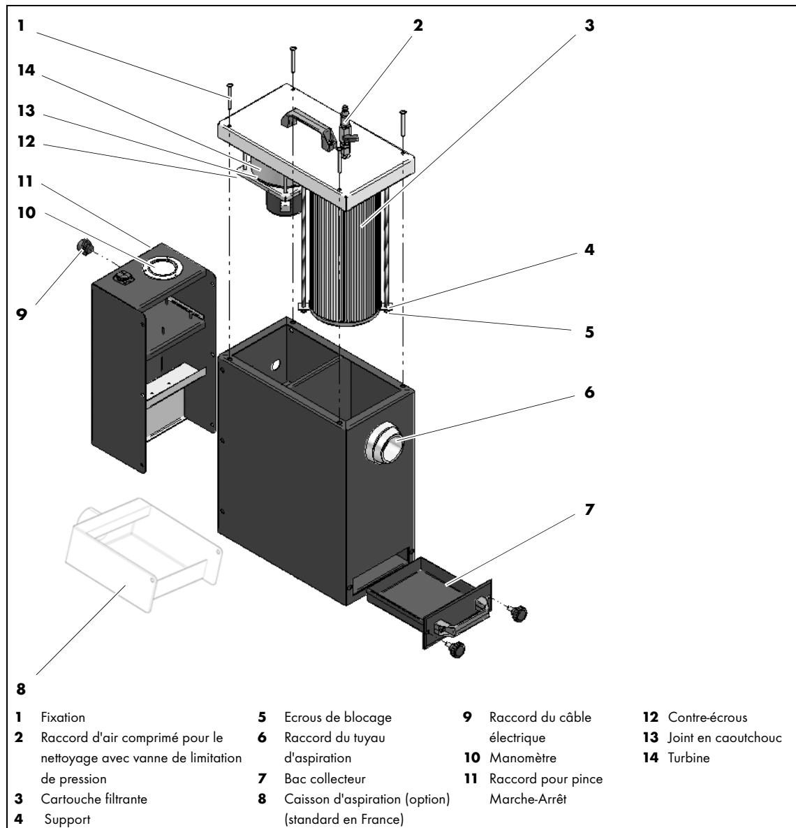
Fig. 2 Description du fonctionnement
