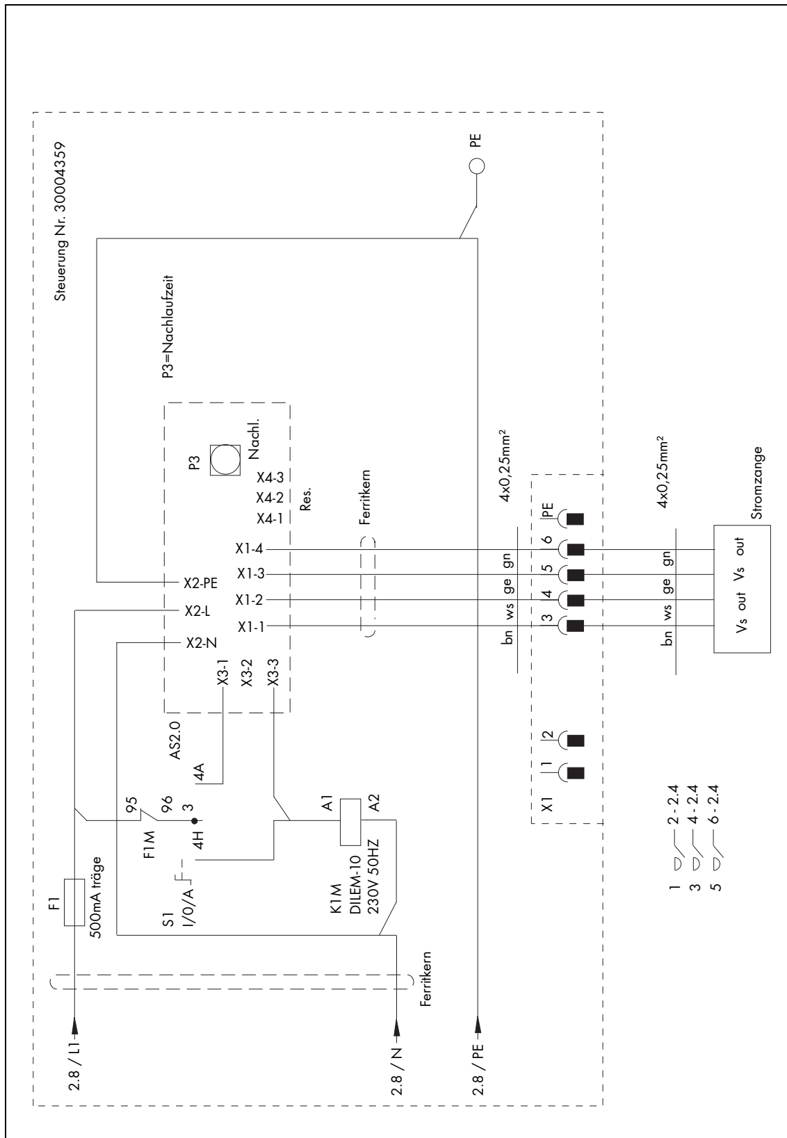
Abb. 7 Elektro-Schaltplan (7-poliger Anschluss)
