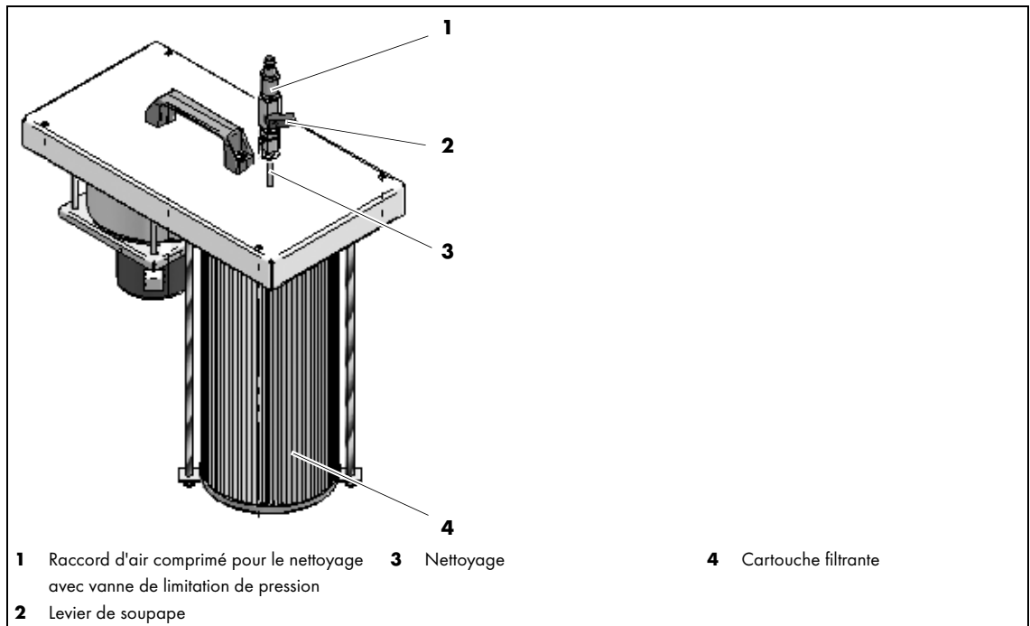
Fig. 3 Nettoyage de la cartouche filtrante
