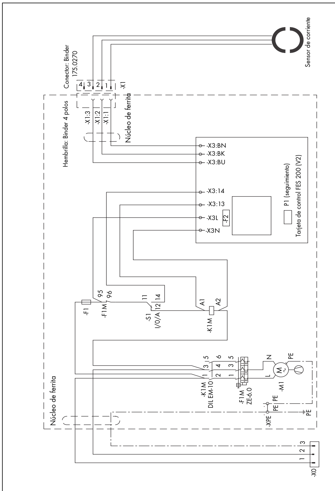
Fig. 8 Esquema de las conexiones eléctricas (conexión de 4 polos)
