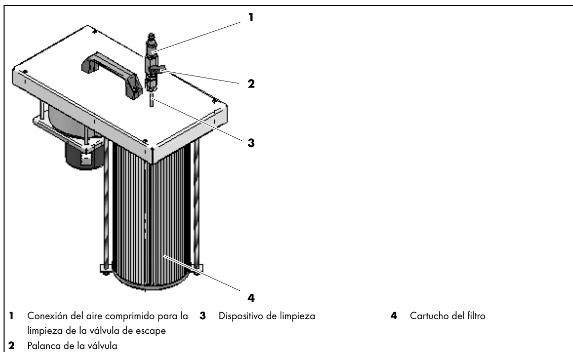
Fig. 3 Limpieza del cartucho del filtro fino
