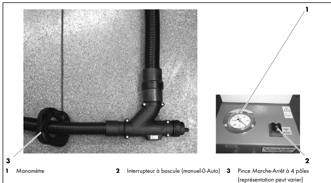
Fig. 5 Pince Marche-Arrêt
