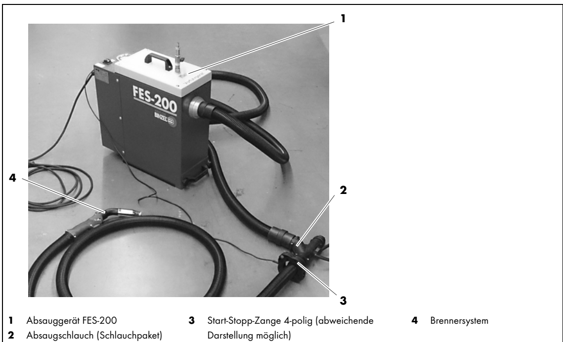
Abb. 4 Inbetriebnahme
