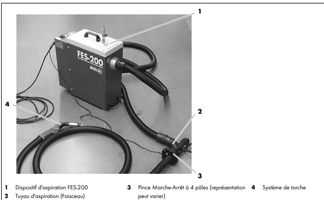
Fig. 4 Mise en service
