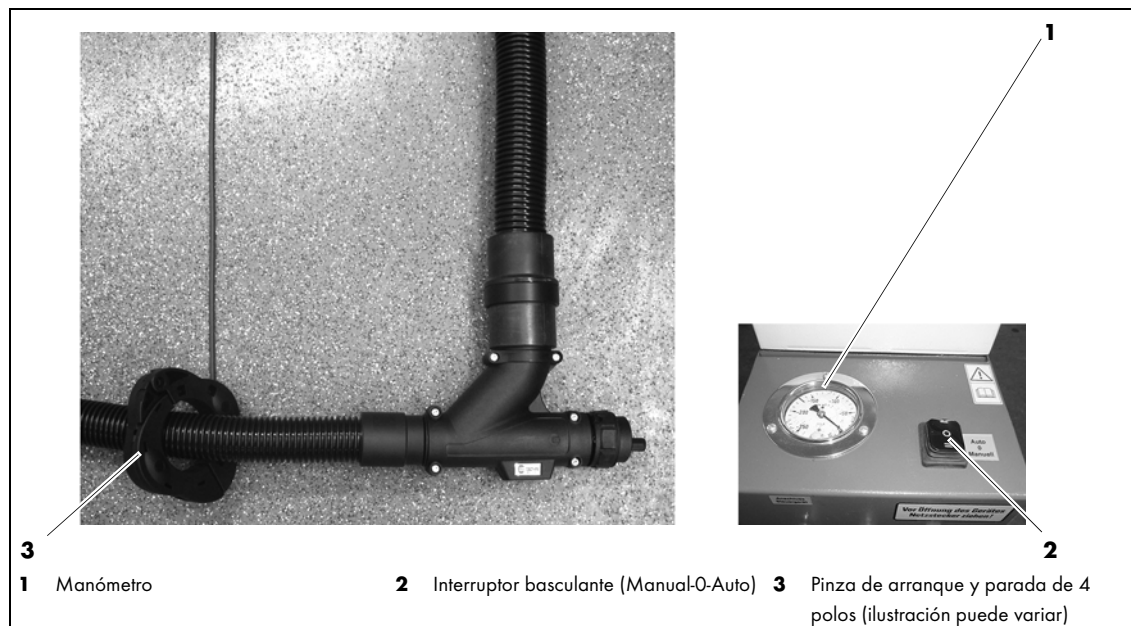
Fig. 5 Pinza de arranque y parada
