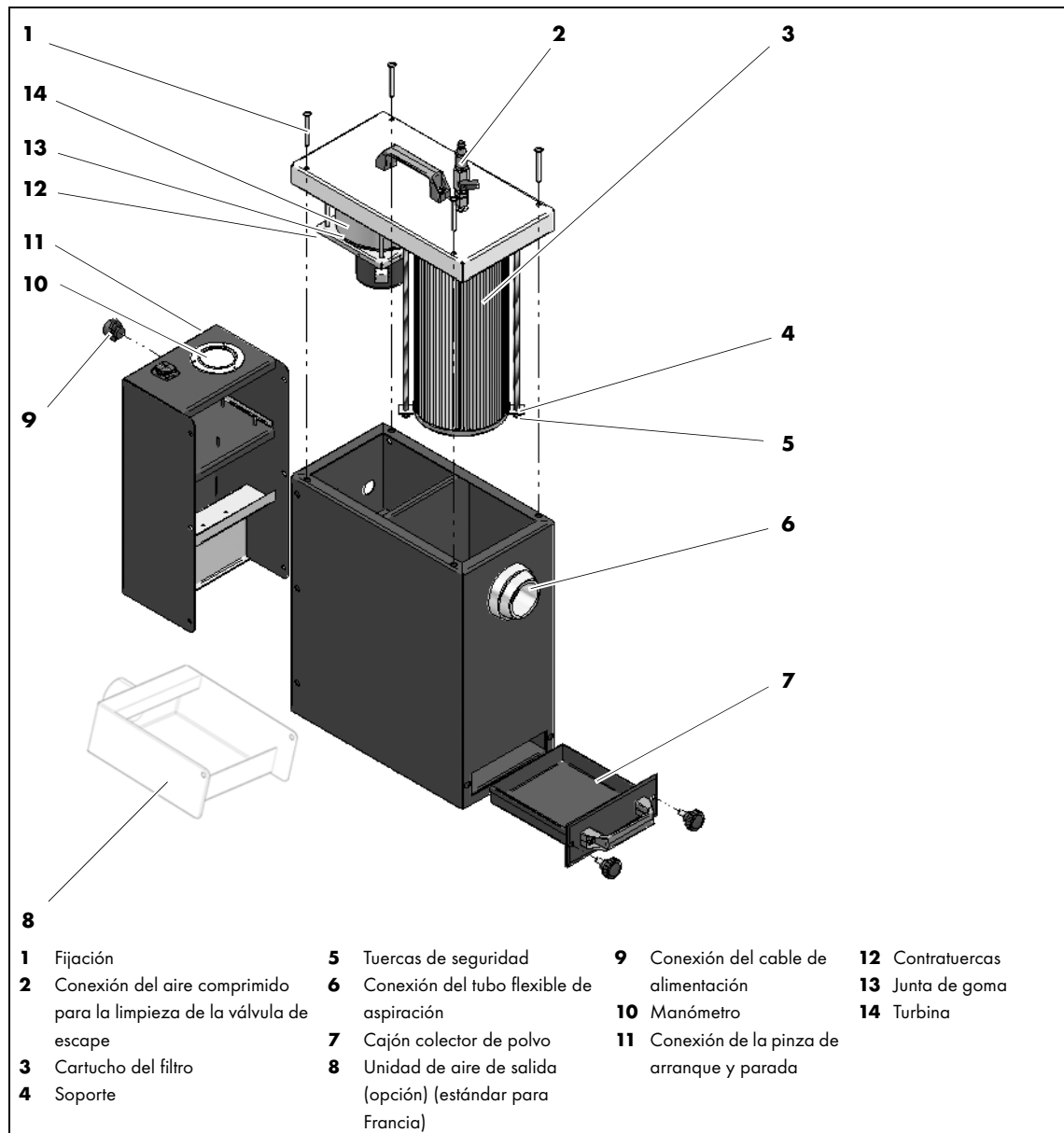
Fig. 2 Descripción del funcionamiento
