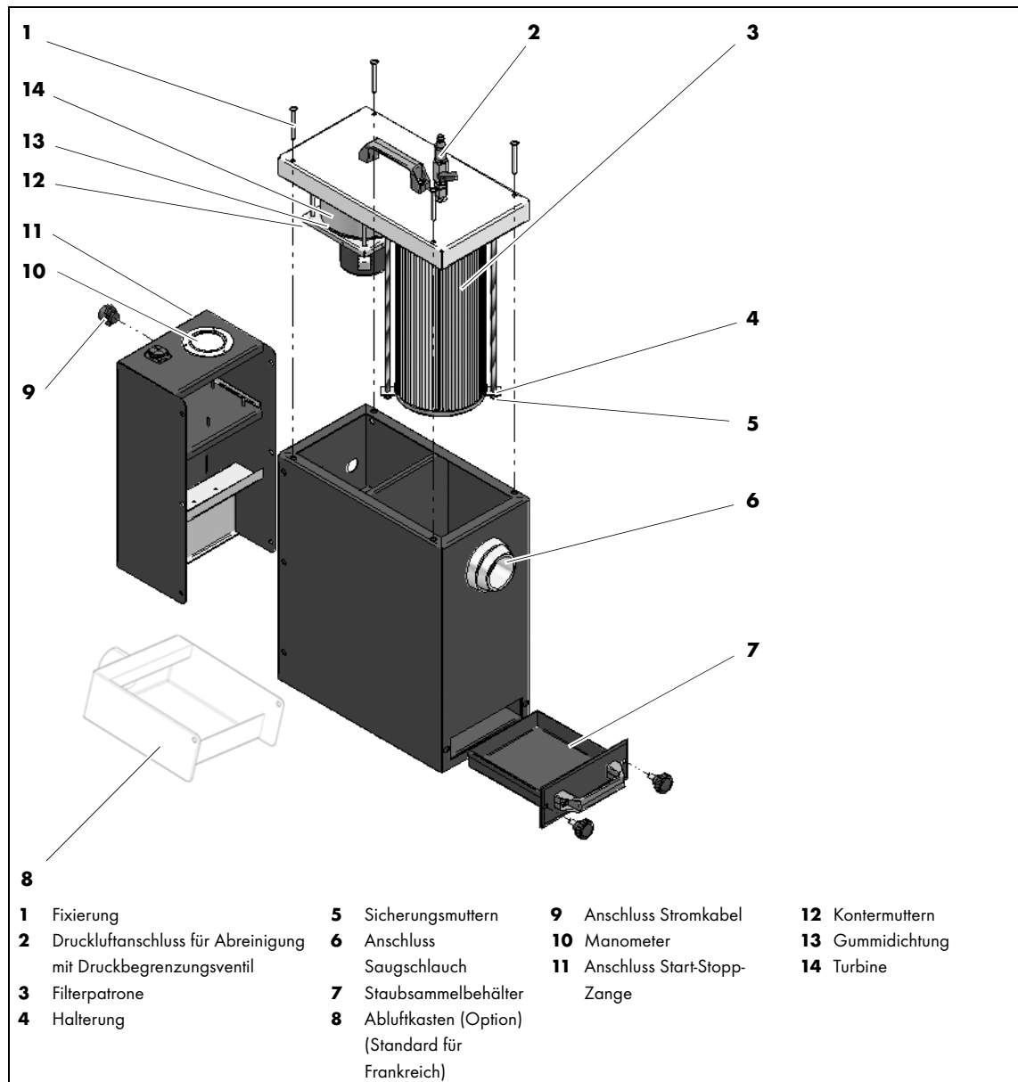
Abb. 2 Funktionsbeschreibung
