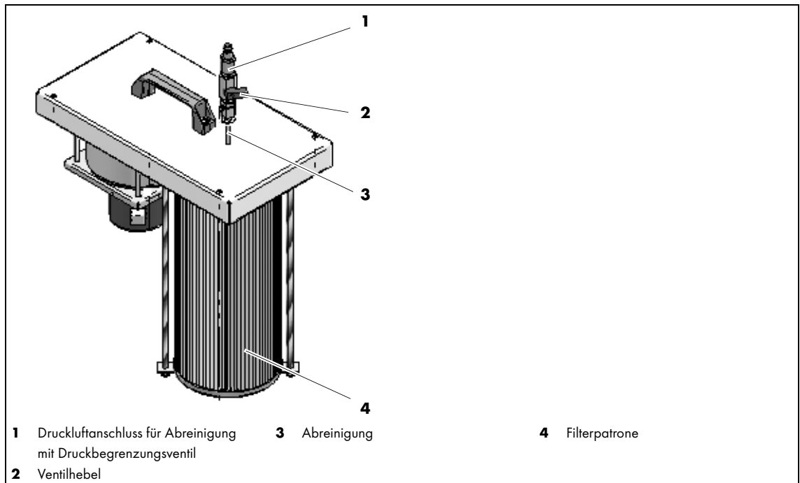
Abb. 3 Abreinigung der Feinfilterpatrone
